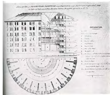
ベンサムによる 一望監視装置 の設計図(1843年)
